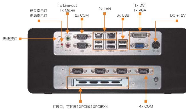
BIS-6595B接口
