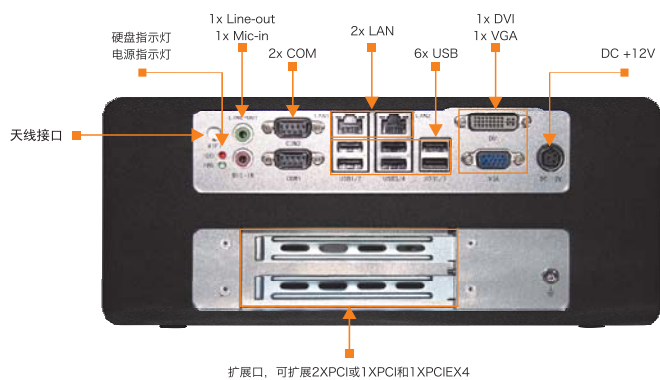
BIS-6595A接口
