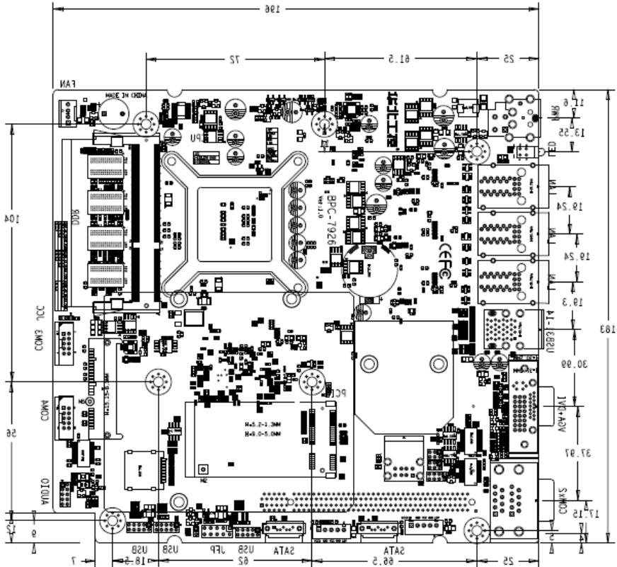
BPC-7926 接口位置和尺寸图
