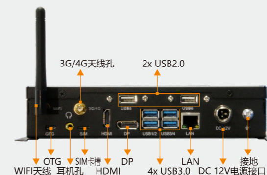
后面板接口
